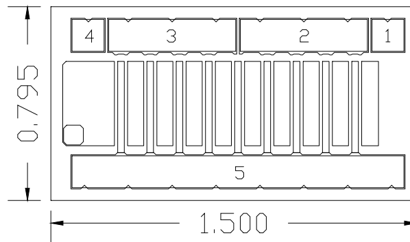
正视图
