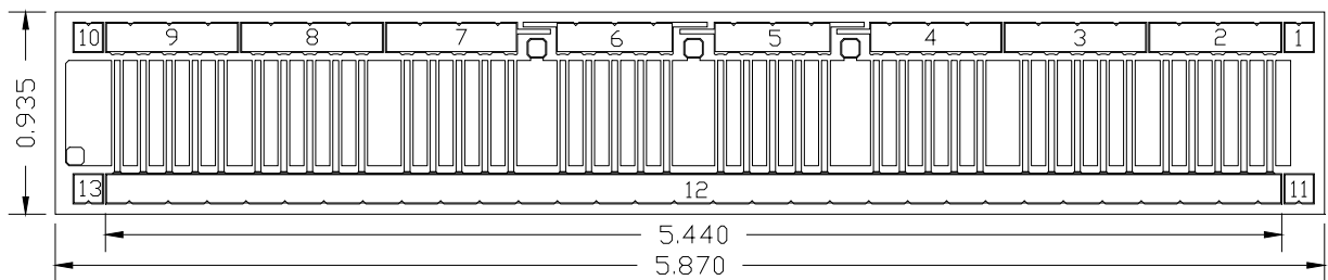
正视图
