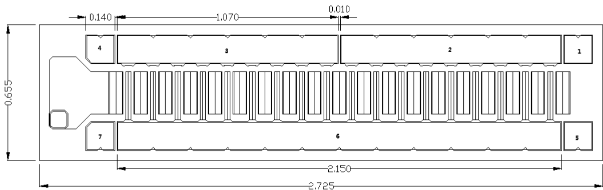
正视图
