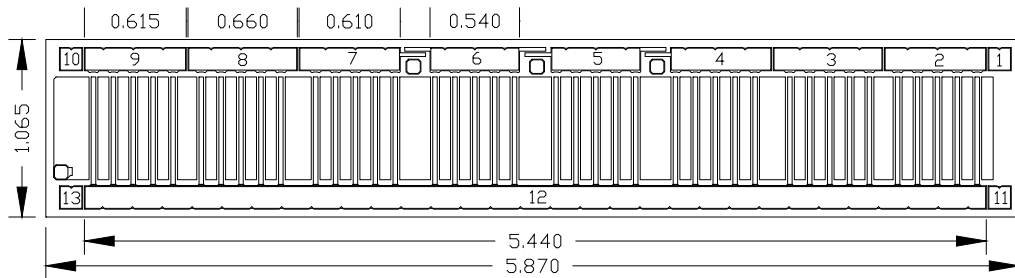
正视图
